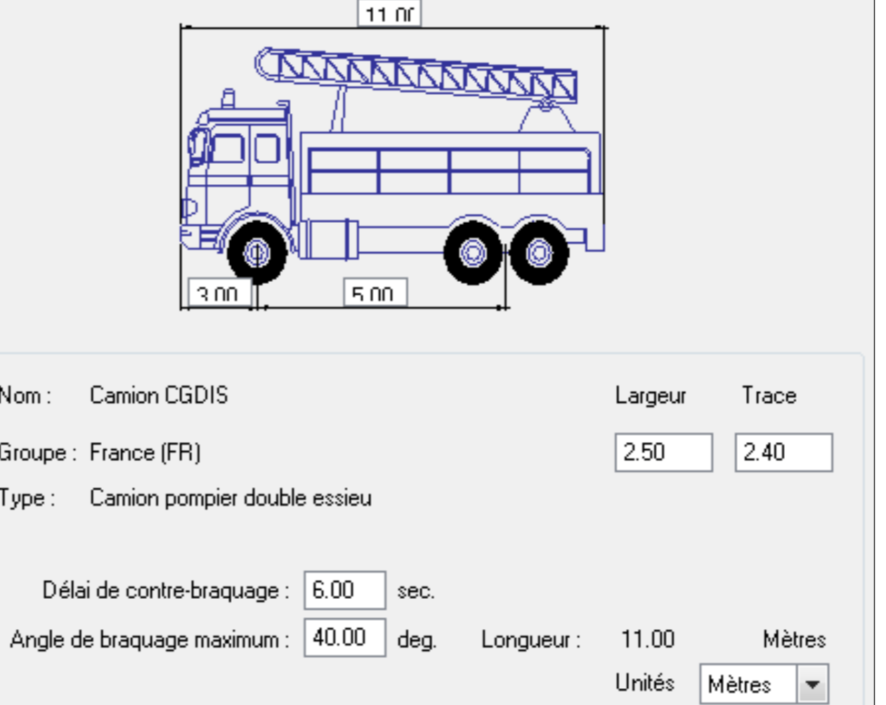
Dimensions camion-échelle CGDIS (Hors échelle)
