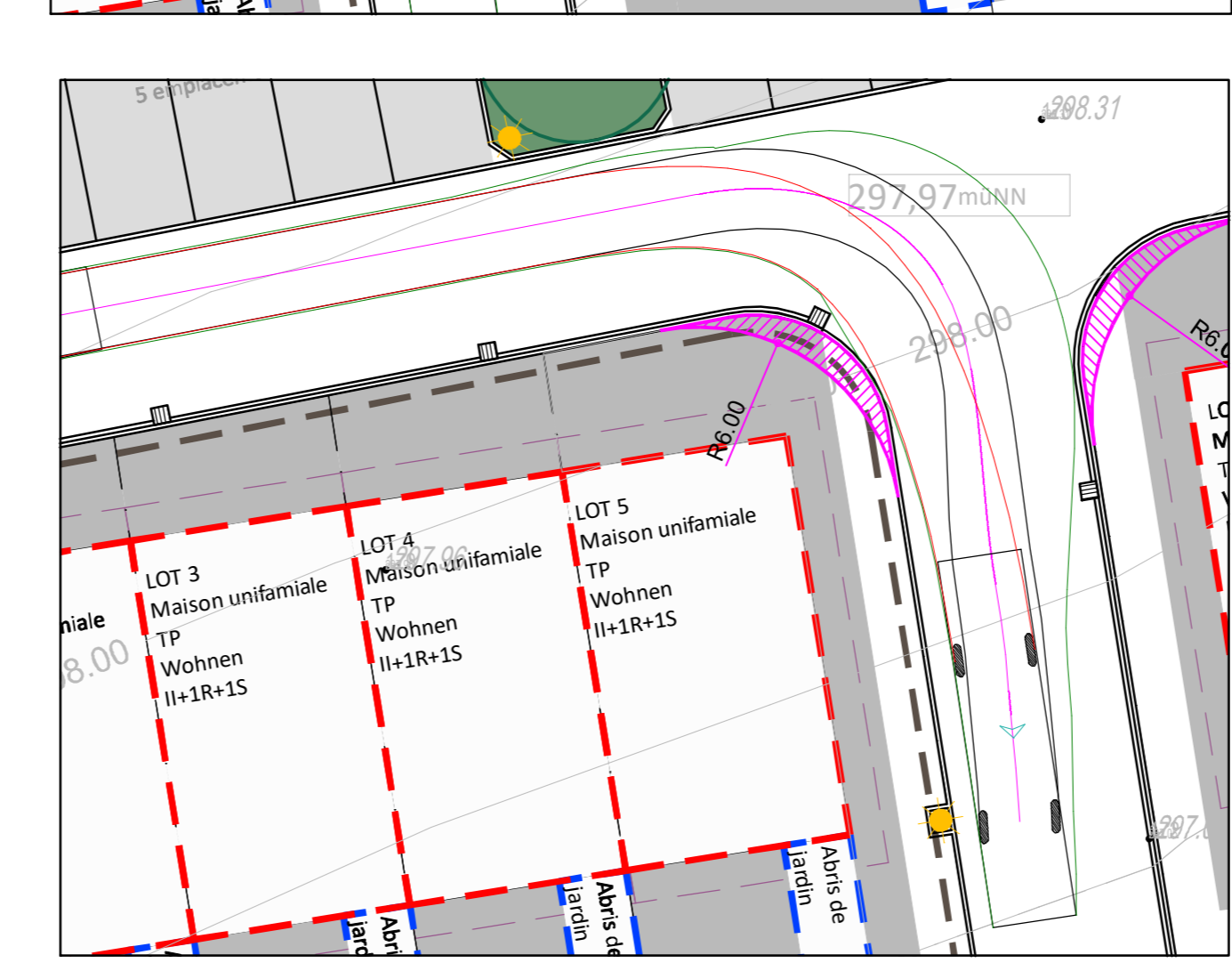
Dimensions camion-échelle CGDIS (Hors échelle)
