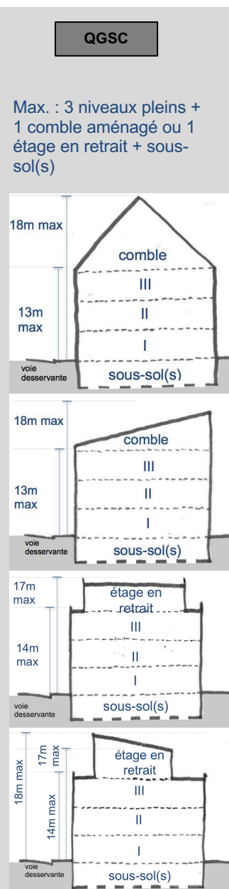
Fig. 30 : Hauteurs des constructions
