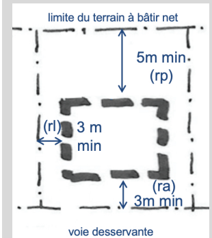
Fig. 35 : Recul antérieur (ra), latéral (rl) et postérieur (rp)
