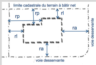
Fig. 43.1 : Immeubles aux angles de rues (plusieurs corps de bâtiment)
