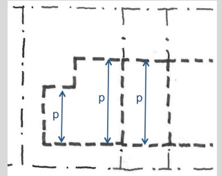
Fig. 5b : Profondeur en cas de maisons accolées (p)
